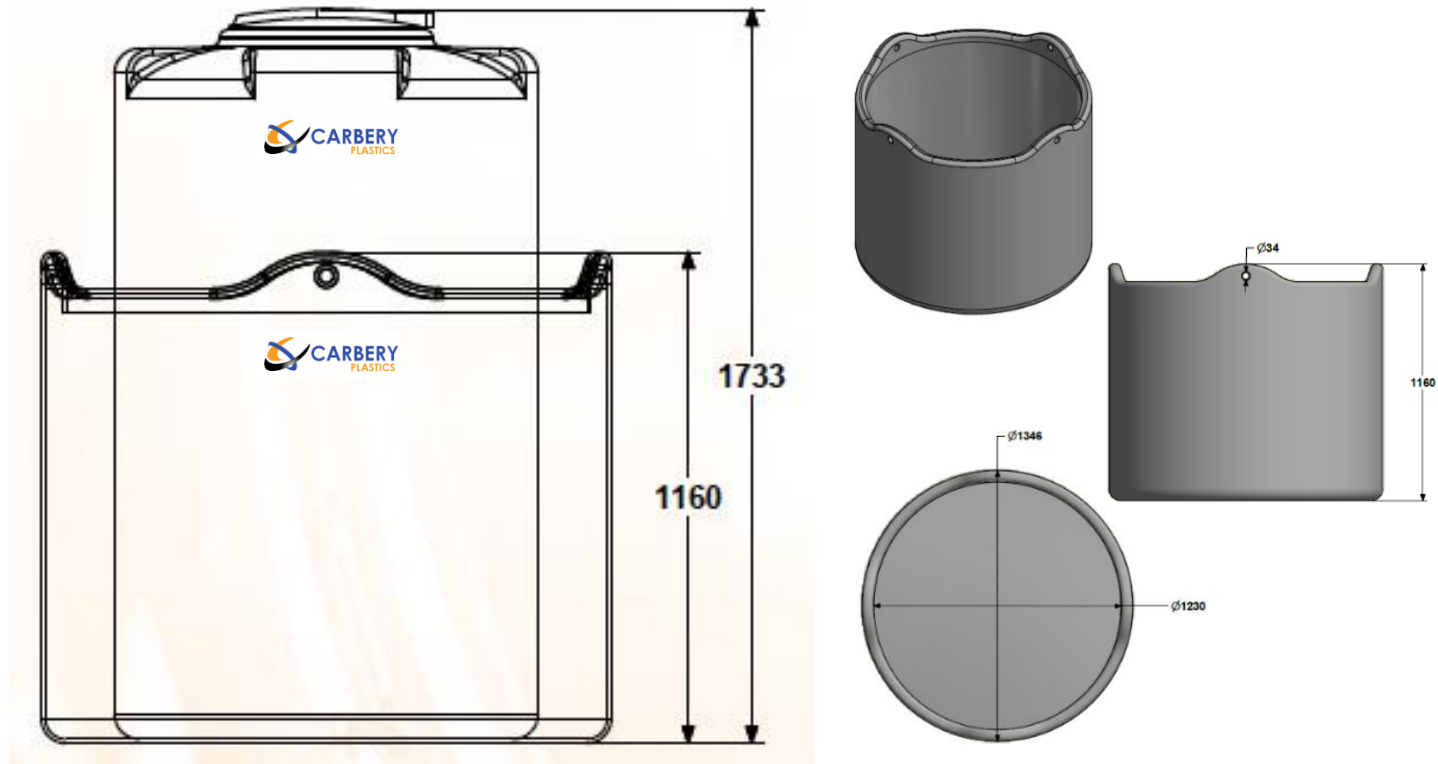
Boven informatie van de 1100 liter tank met bijpassende opvangbak
